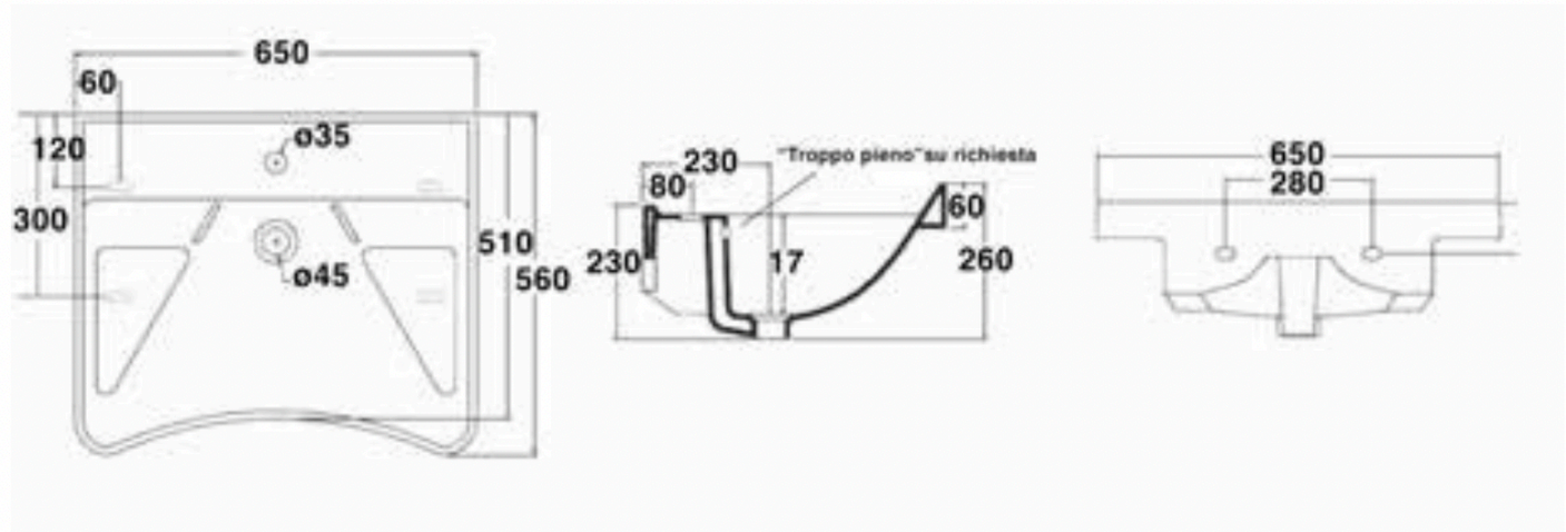
Cod. 1870.00 Lavado Disabili Ergonomico 650x560x230 In Ceramica Bianco Lucido.
